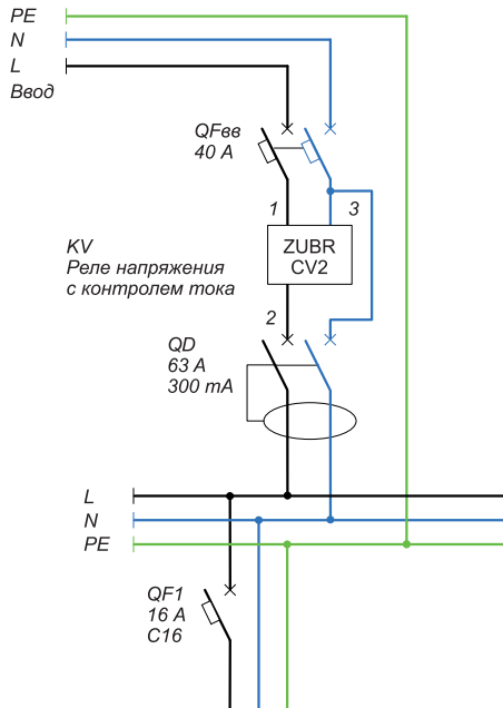
Схема 1. Вариант электрической схемы CV2
