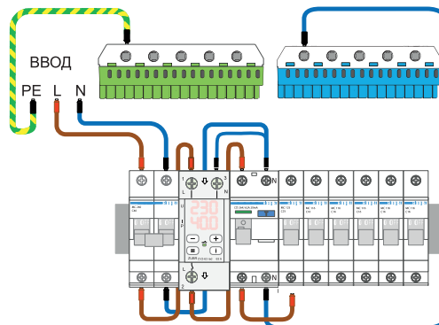
Схема 2. Вариант монтажной схемы CV2
