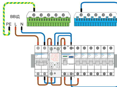
Схема 2. Варіант монтажною схеми CV2
