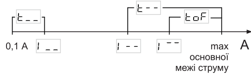
Рисунок 1. Взаємозв'язок меж струму з часом відключення за такими межами
