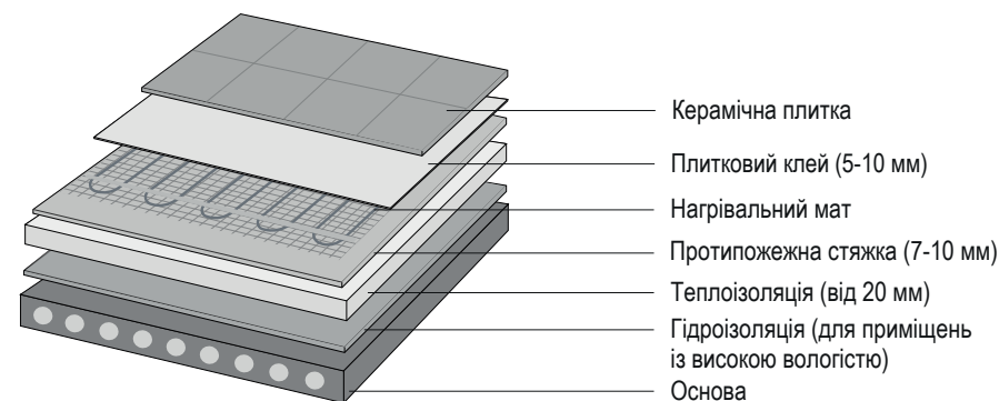
Рис 2. Принцип укладки нагрівального мату
