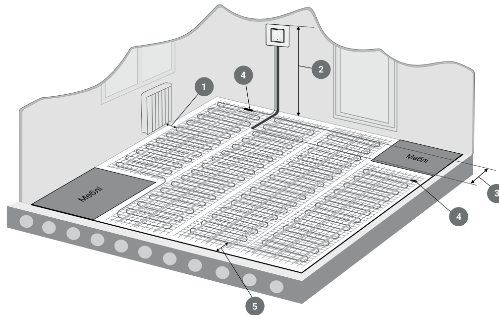
Рис.1 Приклад укладки нагрівального мату
