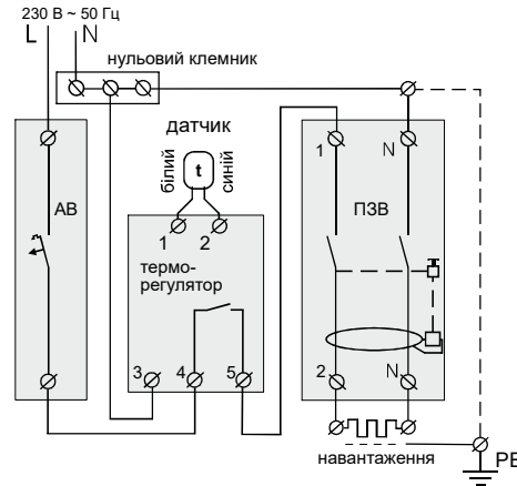
Схема 1. Підключення АВ і ПЗВ
