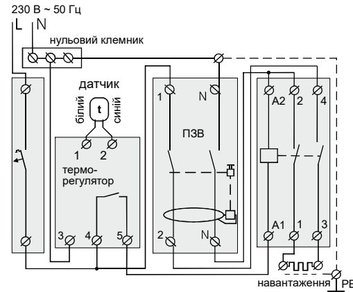
Схема 2. Підключення через магнітний пускач
